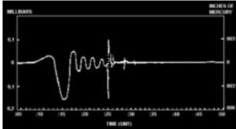
Barogramma che mostra la curva della pressione atmosferica registrata nelle stazioni inglesi nella mattinata del 30 Giugno 1908. (Documento F.J.W. Wipple)
