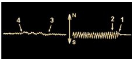
Ingrandimento della registrazione N-S precedente: 1) Inizio oscillazioni alle ore 0h 18,8m TU; 2) Oscillazioni massime alle ore 0h 20,1m; 3) Inizio oscillazioni secondarie alle ore 1h 3,1m; 4) Fine delle oscillazioni secondarie alle ore 1h 9,9m; (Documento I.P. Patechnik)
