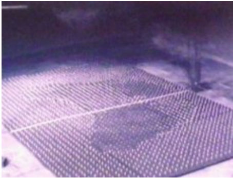
Schema d'abbattimento degli alberi nella forma reale di farfalla, ottenuto in una simulazione di laboratorio presso l'Istituto Schmidt di Mosca.
