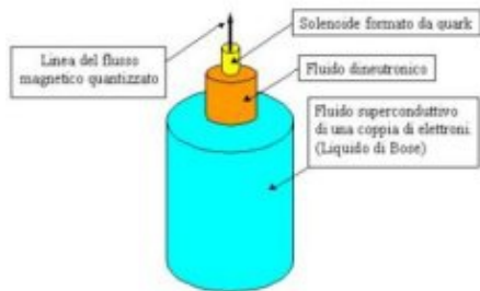
Schema del FLUX secondo Rodionov
