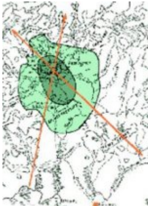
Schema che illustra due possibili traiettorie dell'oggetto esploso sulla Tunguska, proposte dagli scienziati Krinov (traiettoria di destra) e Voznesensky-Astapovich (traiettoria di sinistra).
