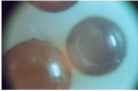
Microsferule ritrovate nel terreno dove si è posato un disco volante, in vicinanza della città di Karaganda (Kazakistan). Era l'anno 1992.
