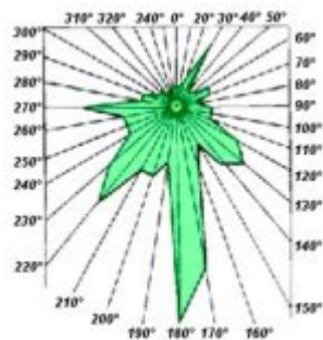
Schema che illustra la quantità dei testimoni in funzione dell'angolo di azimuth della traiettoria, pubblicato da A.N. Dmitriev e V.K. Zhuravlyov nel loro libro del 1984: "Fenomeno del 1908 - Natura delle correlazioni tra la terra e il sole". La maggior parte di loro ha confermato il senso del movimento del corpo che andava da sud a nord.
