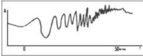
Barogramma, ottenuto sempre il 30 Giugno 1908, dove si possono notare ben due distinti eventi.
