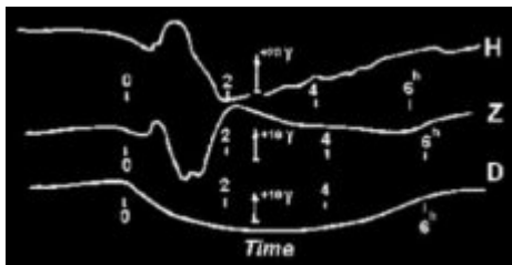
Osservatorio di Irkutsk, 30 Giugno 1908. Il magnetogramma Z riguarda l'esplosione della Tunguska ed è tratto dal libro "Tunguska Marvel" di V.K. Zhuravlyov e F.Yu. Zigel.
