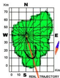
Traiettoria del bolide secondo la teoria di A. E. Zlobin
