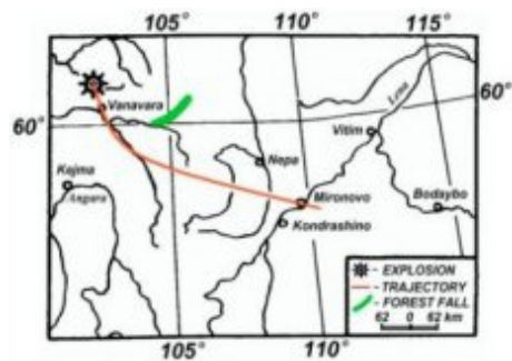
Traiettoria del bolide secondo la teoria di A. E. Zlobin
