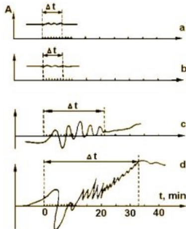
Durata in minuti dell'onda d'aria seguita all'esplosione della Tunguska in funzione della distanza dall'epicentro: a) Irkutsk (distanza 977 Km) - Oscillazioni Nord-Sud; b) Irkutsk - Oscillazioni Est-Ovest; c) Pavlovsk (distanza 3739 Km); d) Londra (distanza 5736 Km); Si può notare che lo spostamento dell'onda d'aria ha avuto una durata proporzionale alla distanza dall'epicentro ed inoltre si possono distinguere sempre quattro eventi di natura esplosiva.
