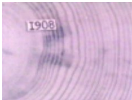
Differenza d'accrescimento di un albero, prima e dopo l'esplosione
