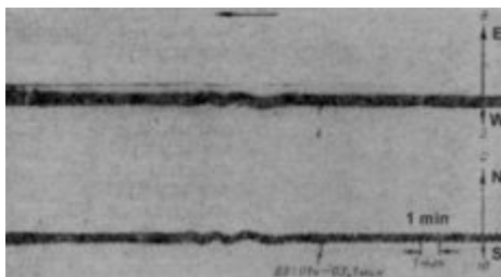
Frammento del sismogramma ottenuto presso l'Osservatorio di Irkutsk. In alto sono rappresentate le oscillazioni E-O e in basso le oscillazioni N-S, le più importanti.
