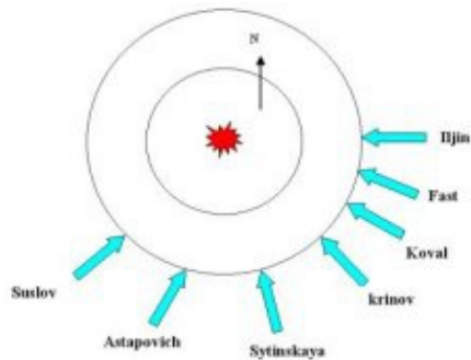
La traiettoria del bolide secondo accreditati studiosi del caso Tunguska
